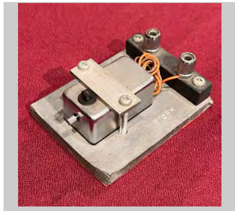
Lot.11 最低入札価格 ￥100,000 トランデューサー 1980年代 日本 10cm シェルマン アンプのスピーカ端子とつなぎ、振動子にサウンドボックスの針先を乗せることで、蓄音器をスピーカーとして使うアダプター 8Ω *別途モノラルアンプ、スピーカーケーブルをご用意ください 経年によるクモリ、使用感あり
